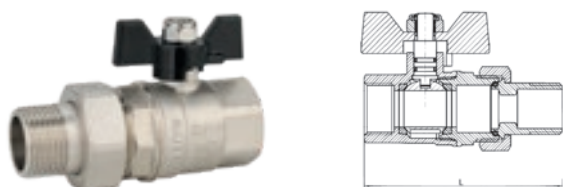
Кран шаровой ВН/НР "бабочка" с разъёмным соединением
