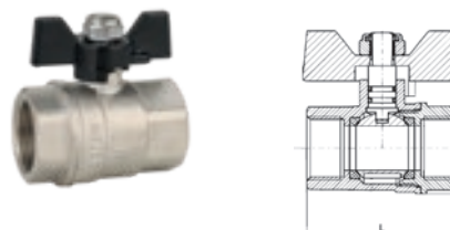
Кран шаровой ВН/ВН "бабочка"
