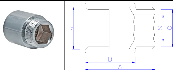
VTr.198.C Удлинитель хромированный В-Н
