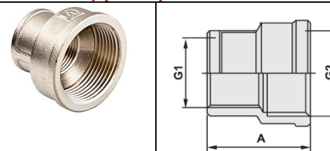
VTr.240 Муфта переходная В-В
