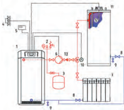
Рис. 8. Гидравлическая схема подключения котла к системе отопления и ёмкостному водонагревателю с разделительным клапаном
