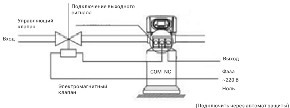
Рис. 10 Подключение электромагнитного клапана на входе
