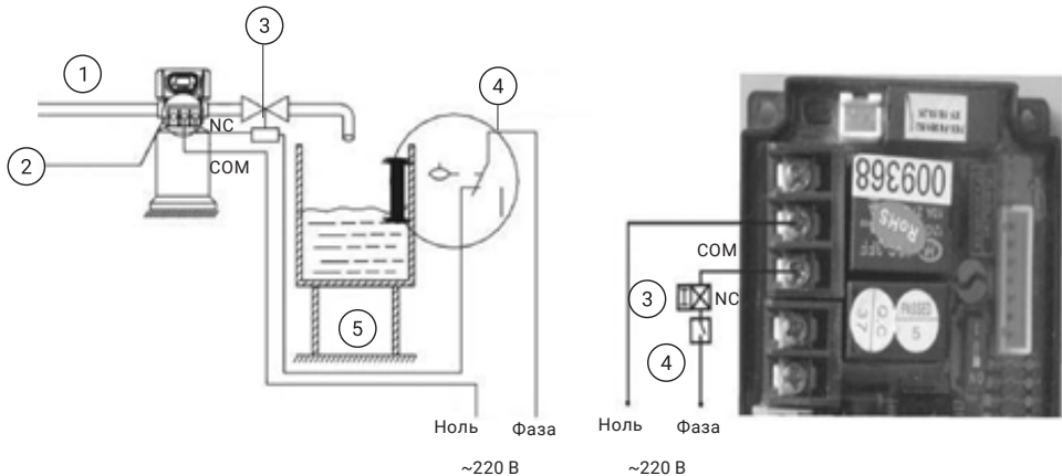
(Подключить через автомат защиты)
